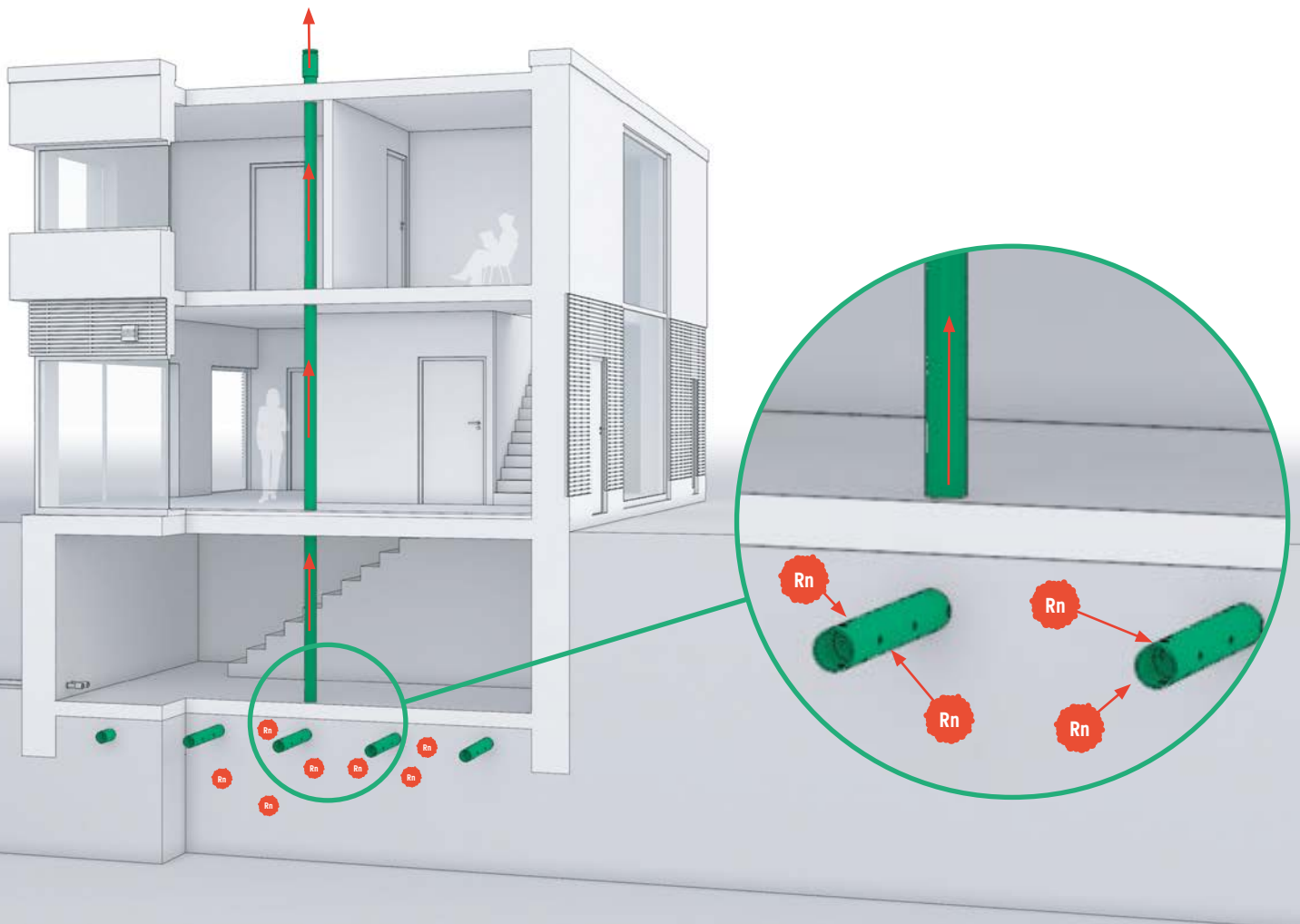
Abb. 7.17: Bodenentlüftung unter der Gebäudesohle mittels Drainagesystem
