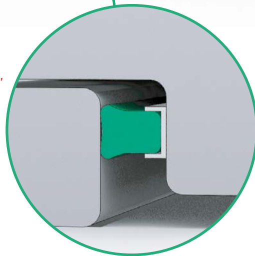
Abb. 7.12: Türschwellen mit Dichtungsprofilen, auch für den nachträglichen Einbau
