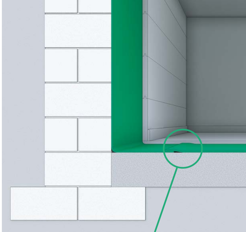
Abb. 7.3: Raumseitige Abdichtung mit Dichtungsbahnen
