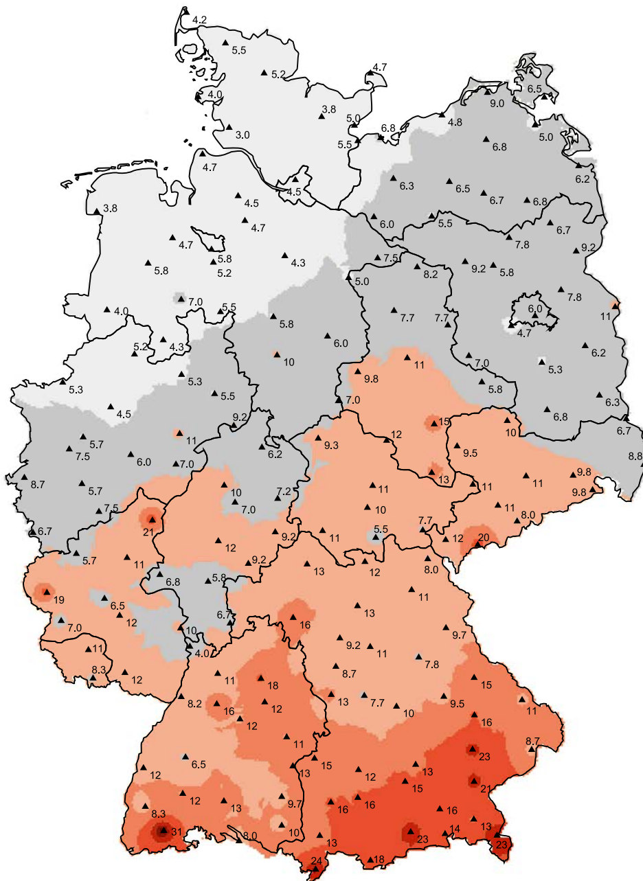
Abb. 3.3: Radon-222-Konzentration in der bodennahen Atmosphäre in Bq/m 3
