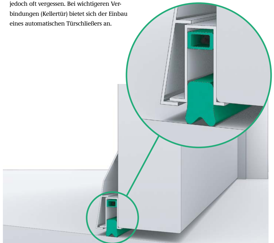
Abb. 7.13: Bewegliche Anpress-Schwelldichtung
