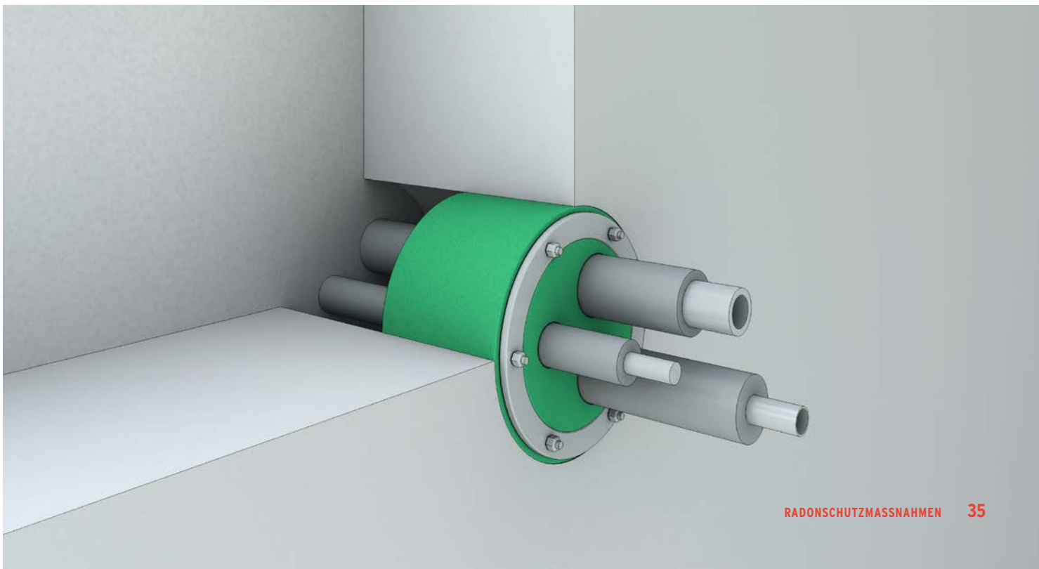
Abb. 7.9: Fachgerechte Abdichtung der Dichtungsbahnen bei Durchstoßungen
