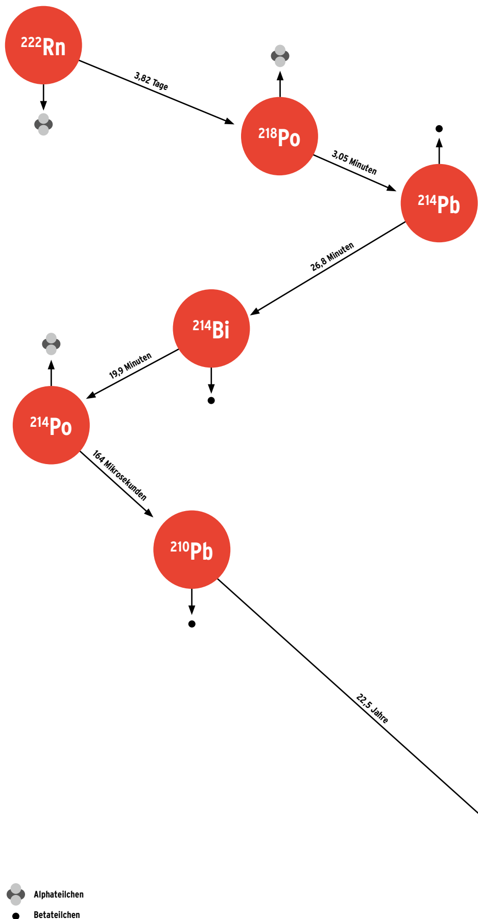
Abb. 1.1: Zerfallsreihe des natürlichen, radioaktiven Isotops Radon-222 mit Halbwertszeiten
